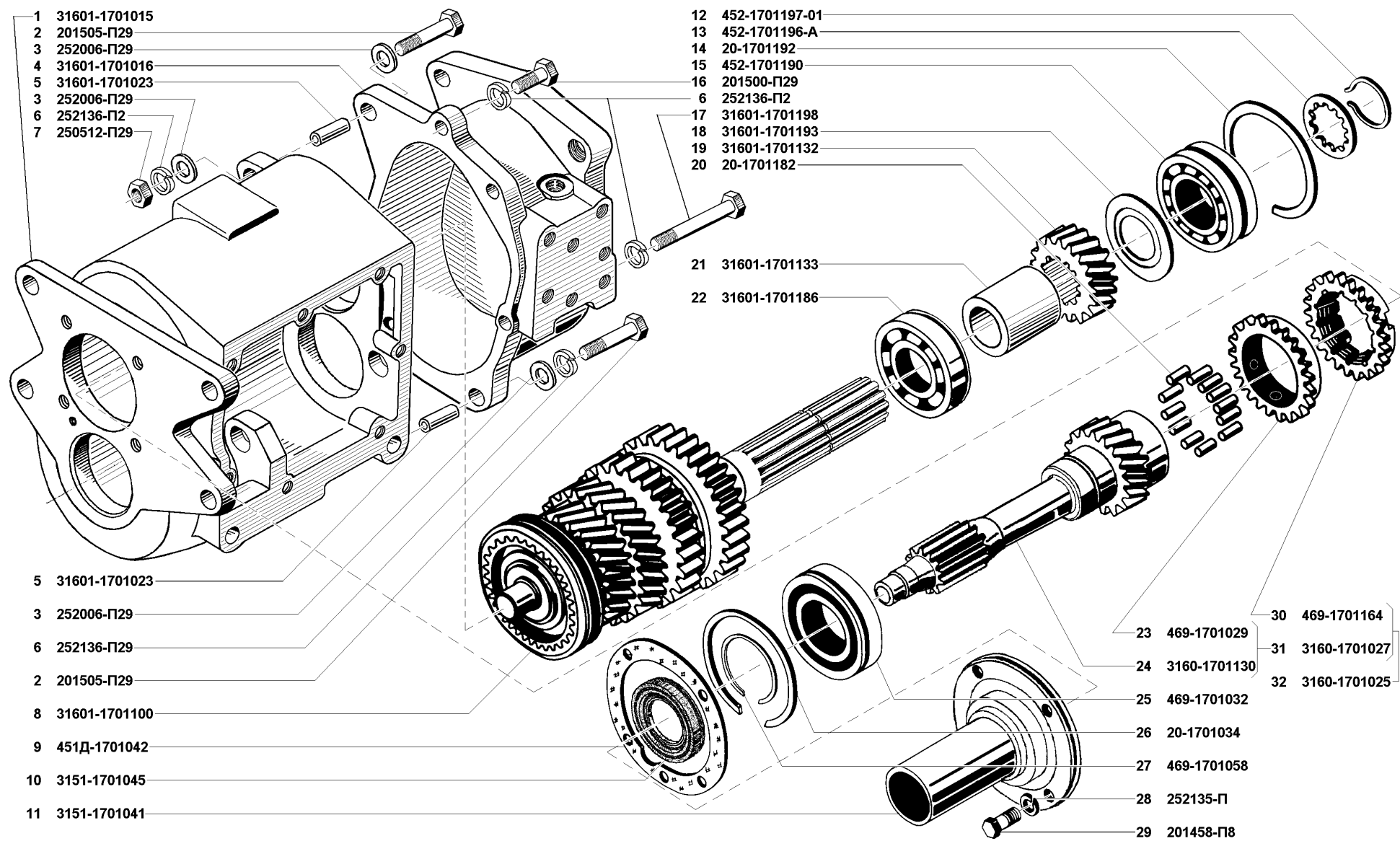
Рис. 51. Коробка передач (1701+)/1
