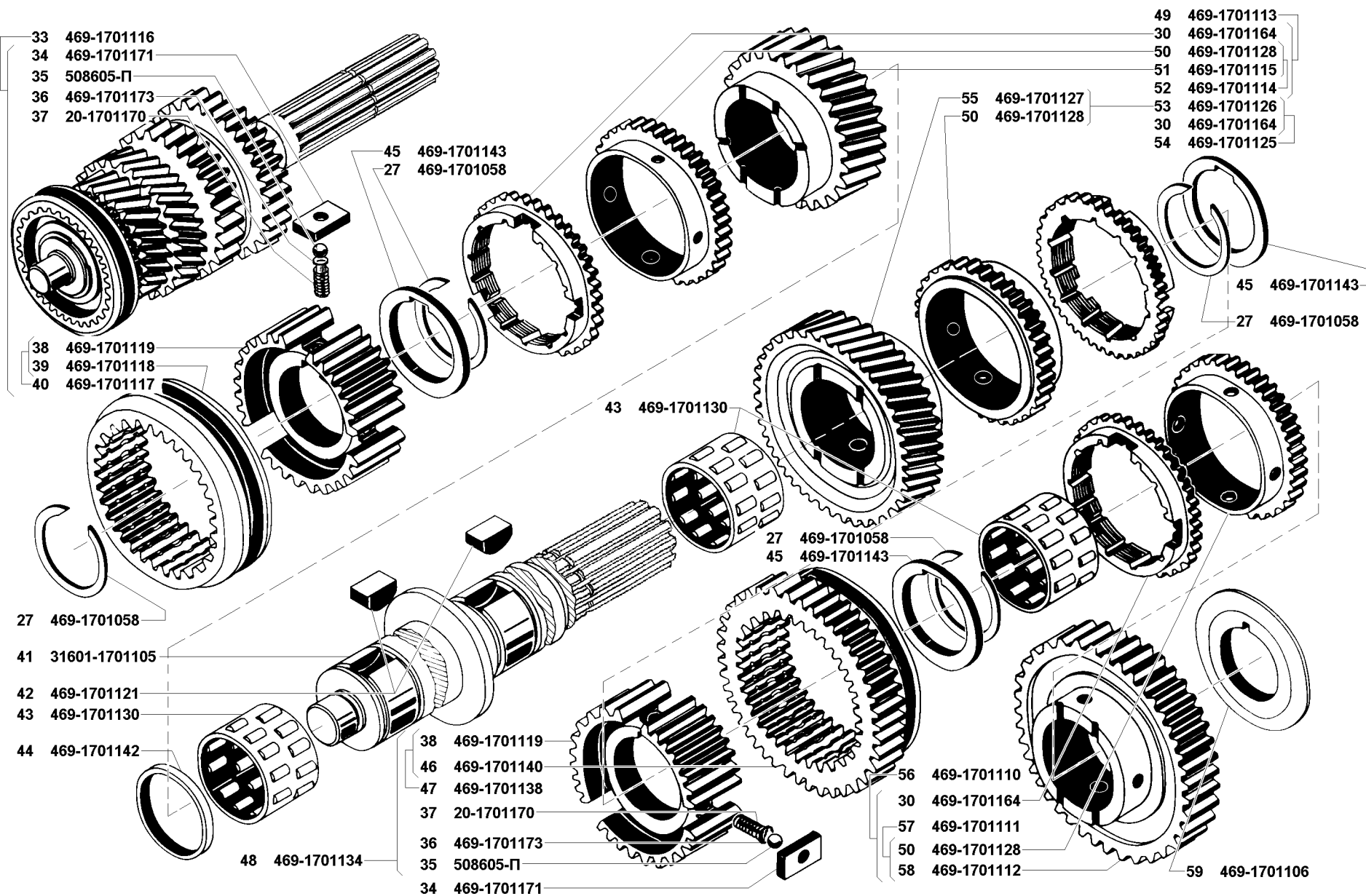
Рис. 52. Коробка передач (1701+)/2
