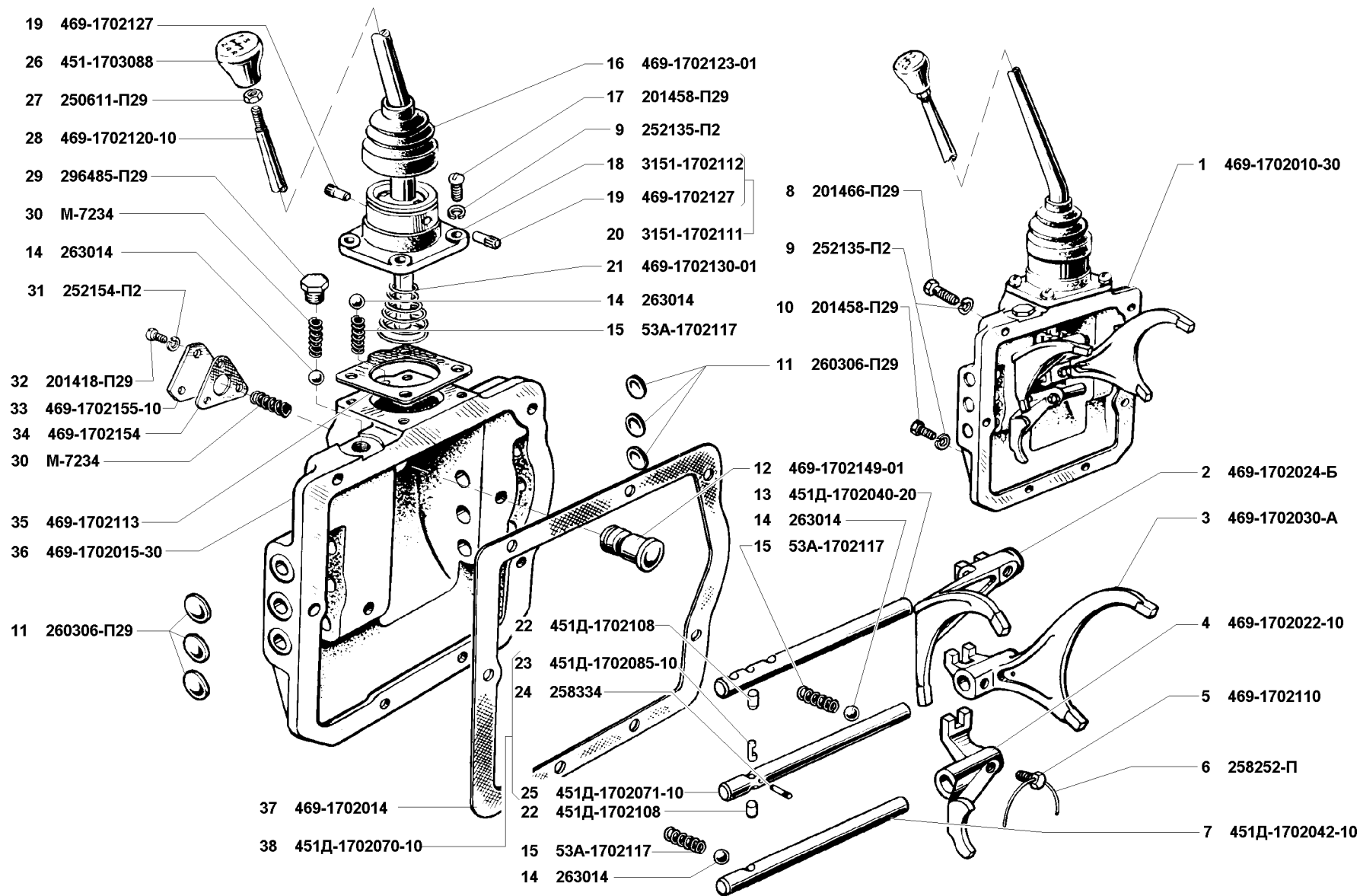
Рис. 50. Механизм переключения передач (1702+)
